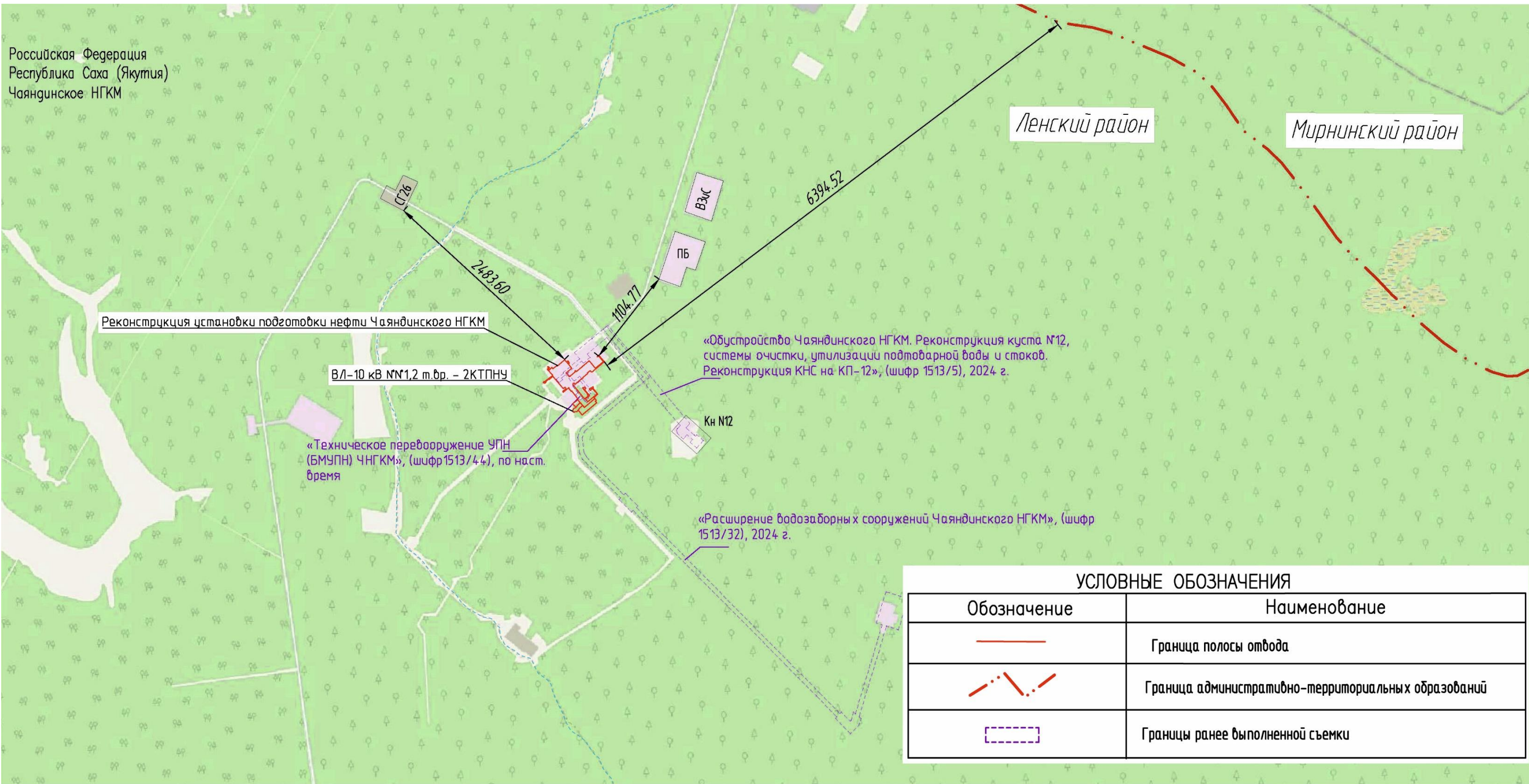
Рисунок 1.1 – Карта-схема размещения проектируемых сооружений
